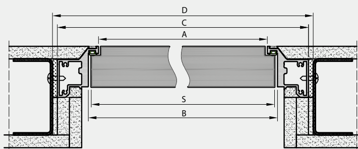
Przekrój poprzeczny drzwi Sara Eco (montaż w ścianie G-K)
