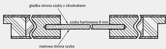
Przekrój poziomy drzwi VETRO B5, B8-B11
