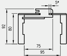
Przekrój ORB 075
