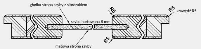
Przekrój poziomy drzwi VETRO A5, A8-A11
