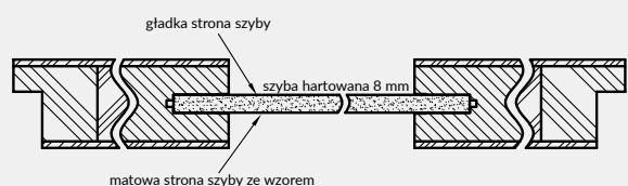
Przekrój poziomy drzwi VETRO A5, A8-A11
