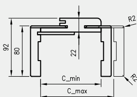
Przekrój ORB 075
