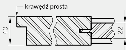
Przekrój poziomy drzwi Elsa
