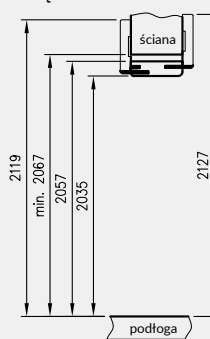
Przekrój pionowy tunelu regulowanego z ką. T80
