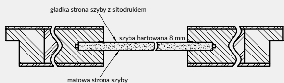
Przekrój poziomy drzwi VETRO A5, A8-A11
