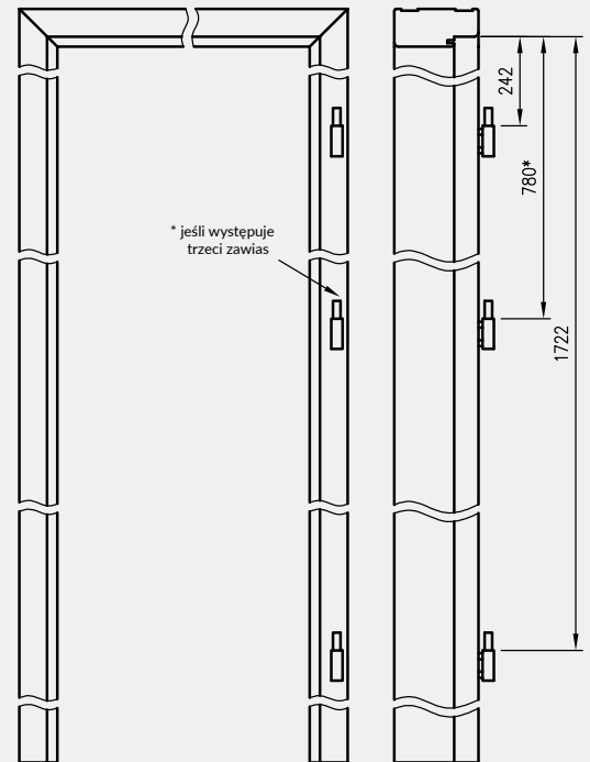
przekrój ościeżnicy prostej SOFT natura
