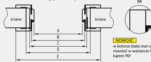
Przekrój poziomy ORB
